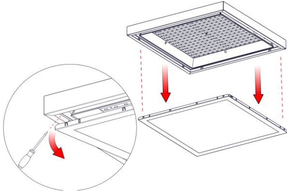
1) Armatürün difüzörü çıkartılır. The armature diffuser is removed.
