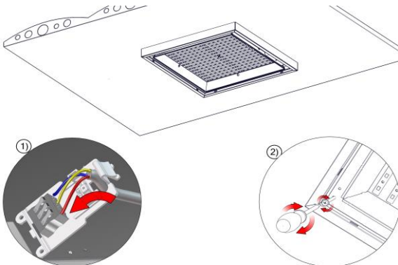
3) Elektrik bağlantısı yapılır askı vidası sıkılır. The electrical screw is tightened.
