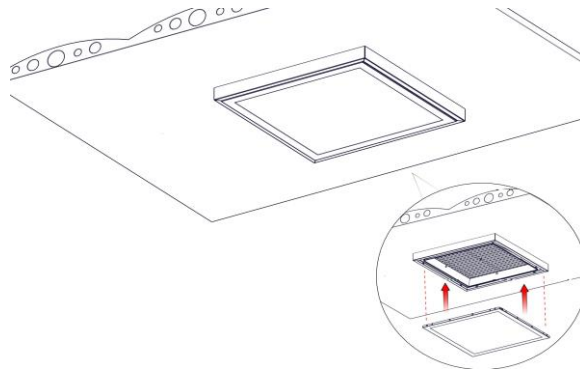
4) Difüzörün gövde ile bağlantısı yapılarak montaj tamamlanır. Assembly is completed by connecting the diffuser to the body.
