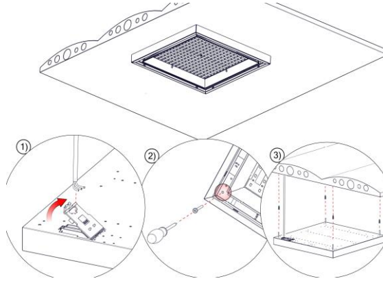
2) Armatürün kablo girişi yapılır tavan montajı için uygun dübeller ile tavana sabitlenir. The armature is fixed to the ceiling with the appropriate anchor for cable entry.
